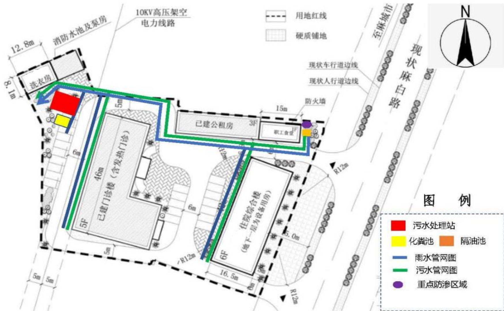
附图5 项目雨污管网图
